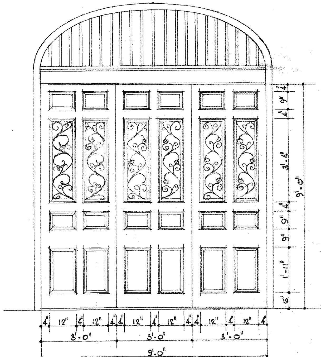
† GATE N o 2 † SCALE 1/2" = 1'-0" †
